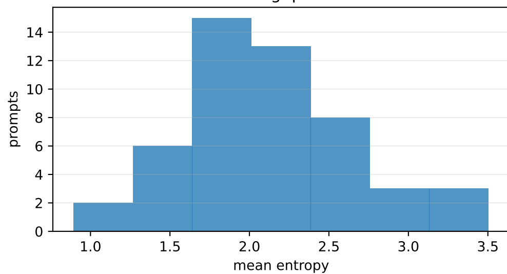
logiqa
