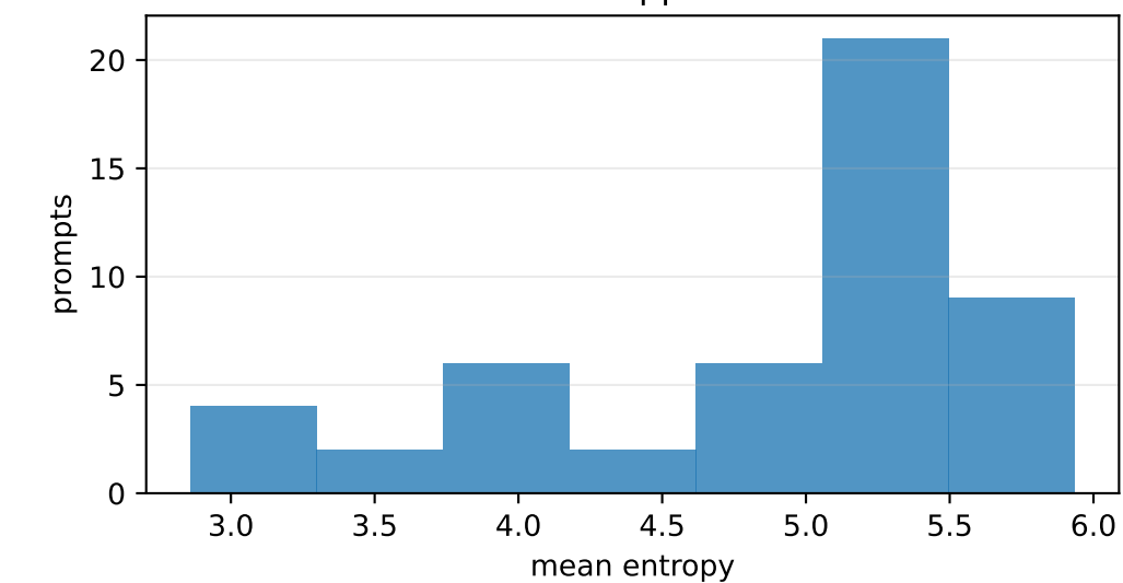
oasst1
