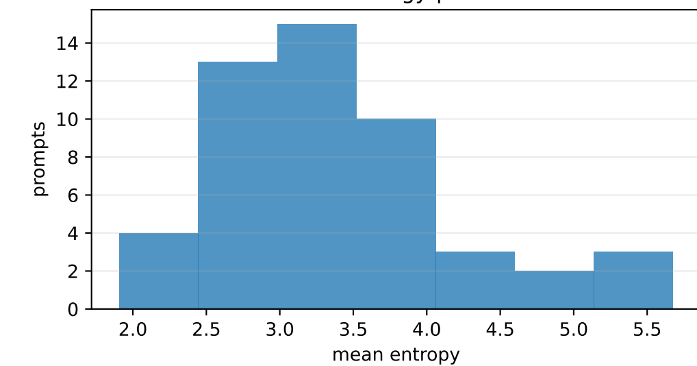
strategyqa
