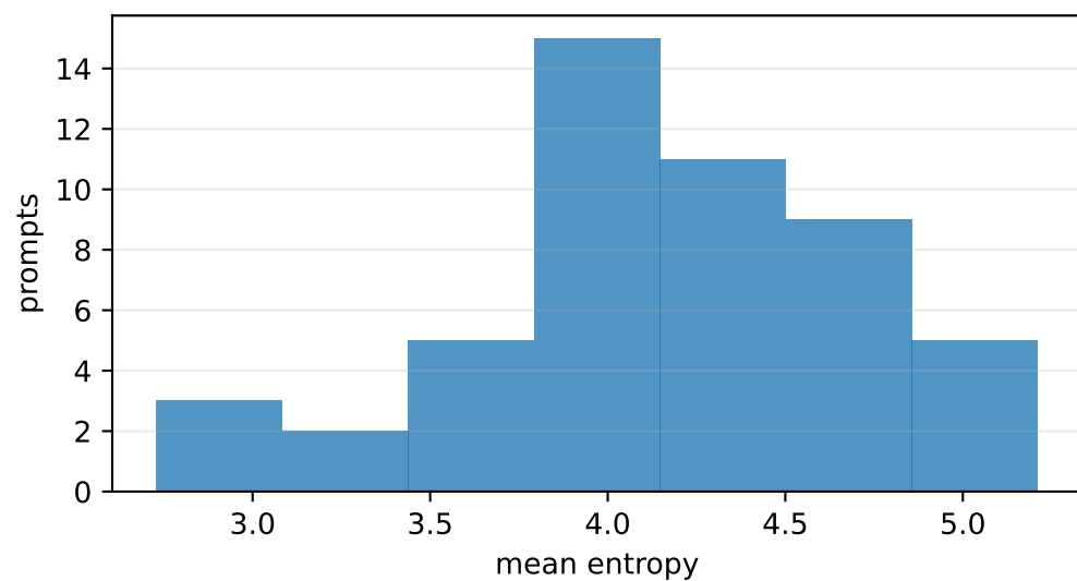
daily_dialog
