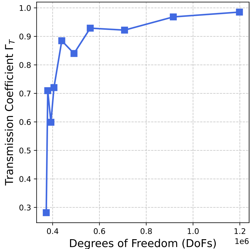
Scattering Parameter Convergence
