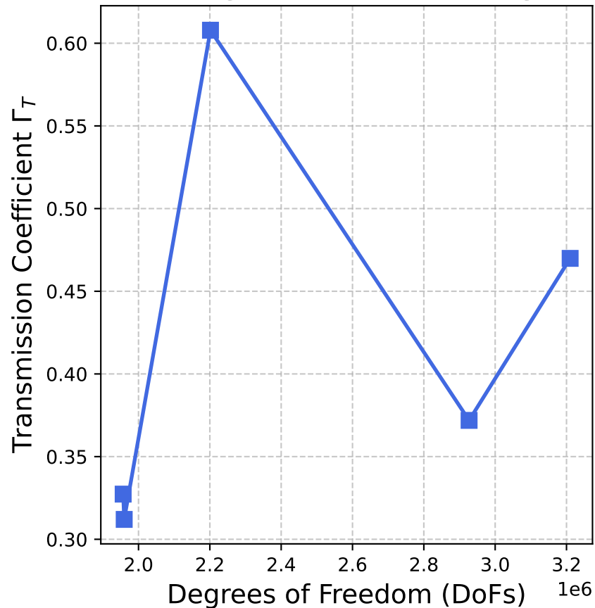
Scattering Parameter Convergence
