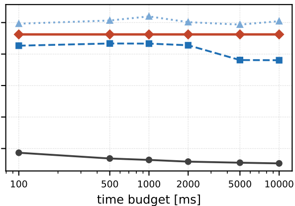
Motzkin
