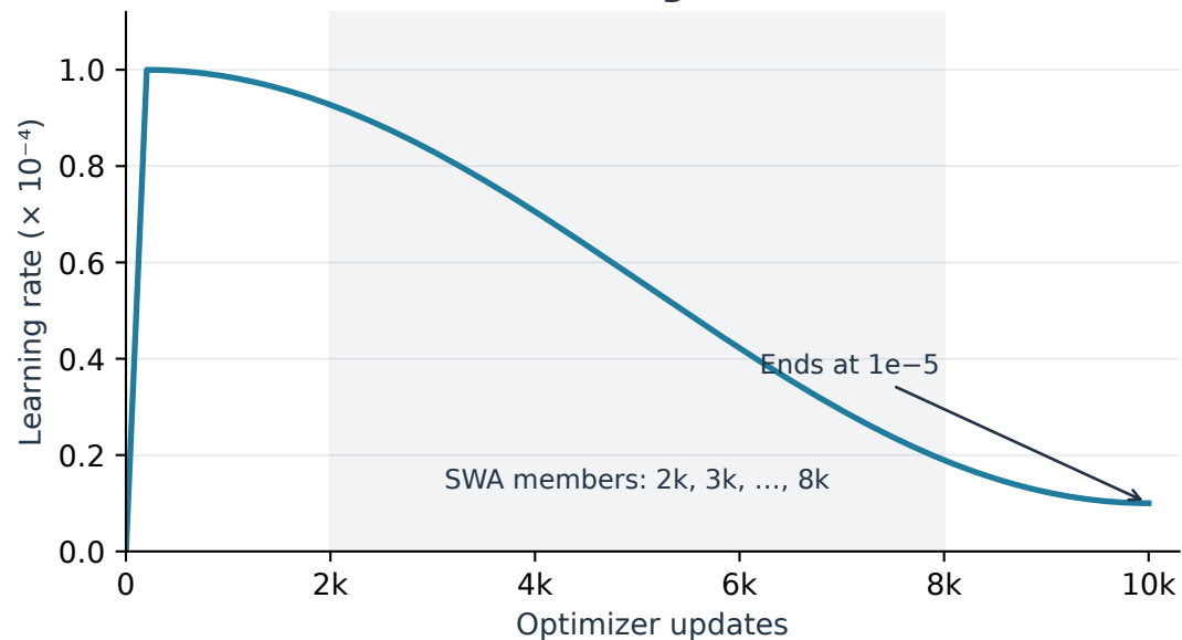
C Actual learning-rate schedule
