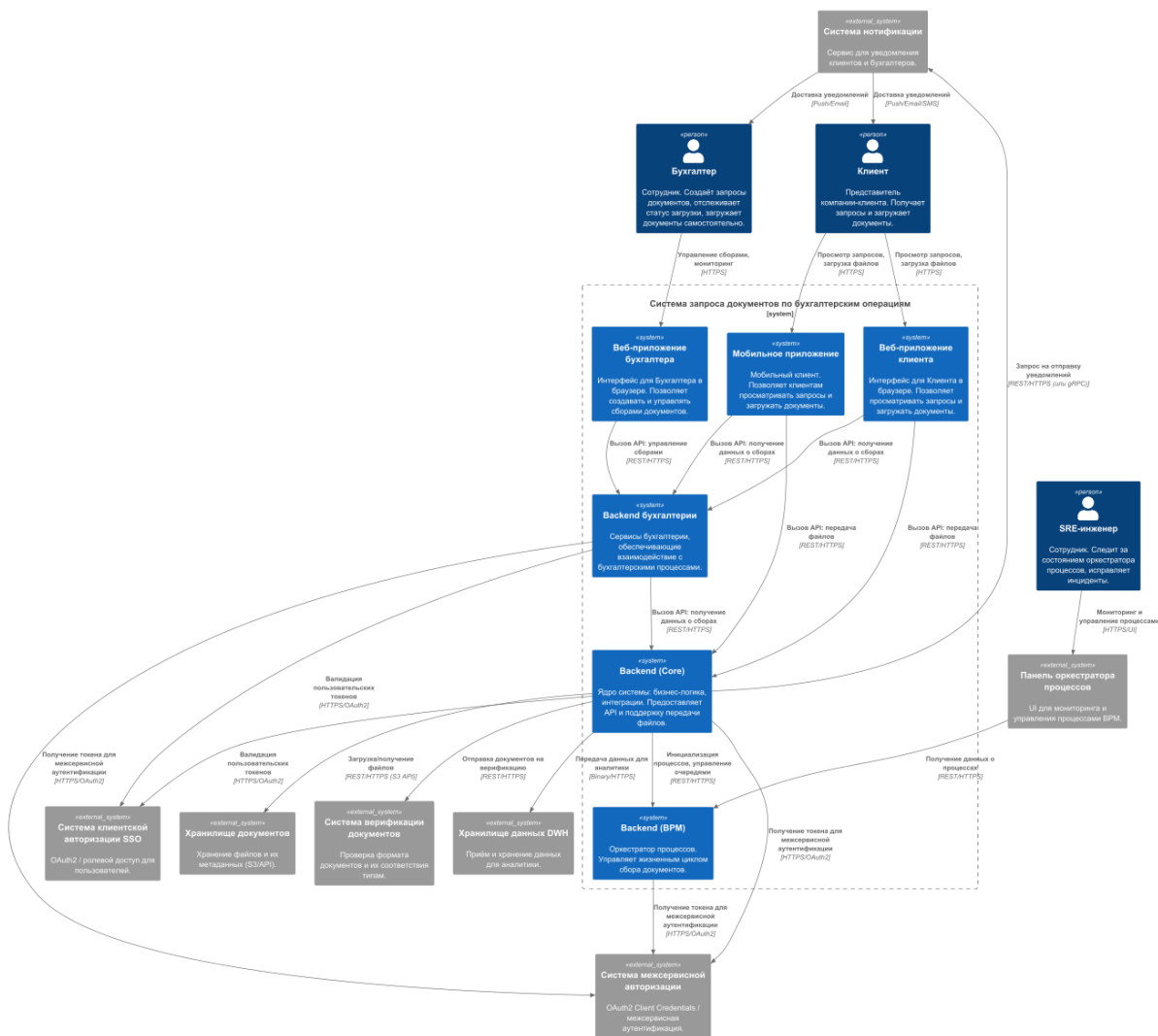
Рисунок 16 – C4-context диаграмма
