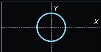
POISSON · ELLIPTIC
