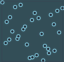
Latin hypercube
