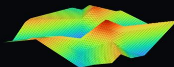
RMSE 0.137
