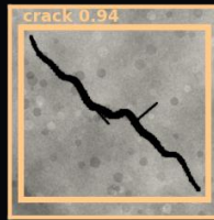
DETECT
