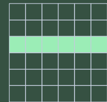
layer norm
