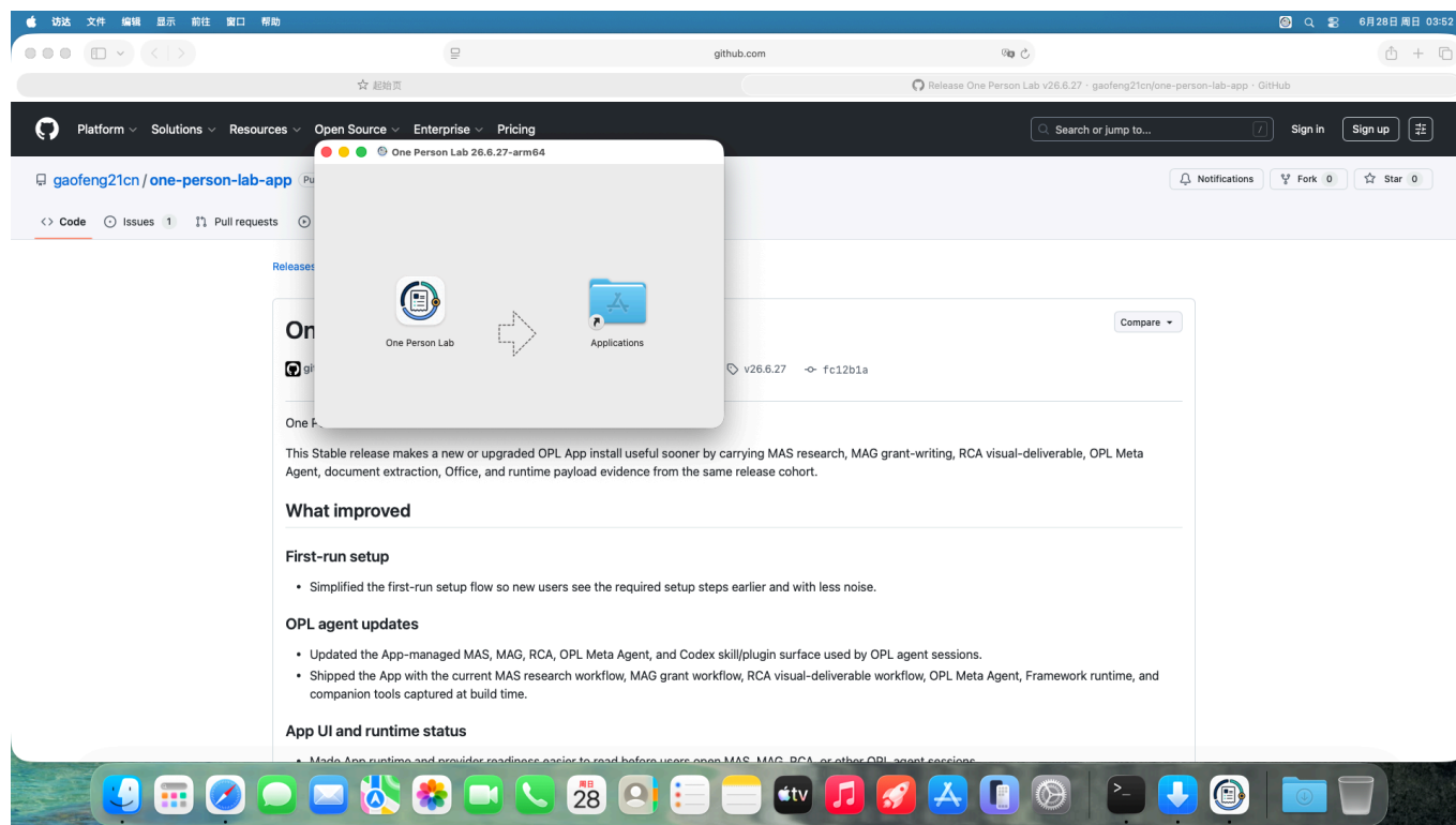
图 2: 安装 App
