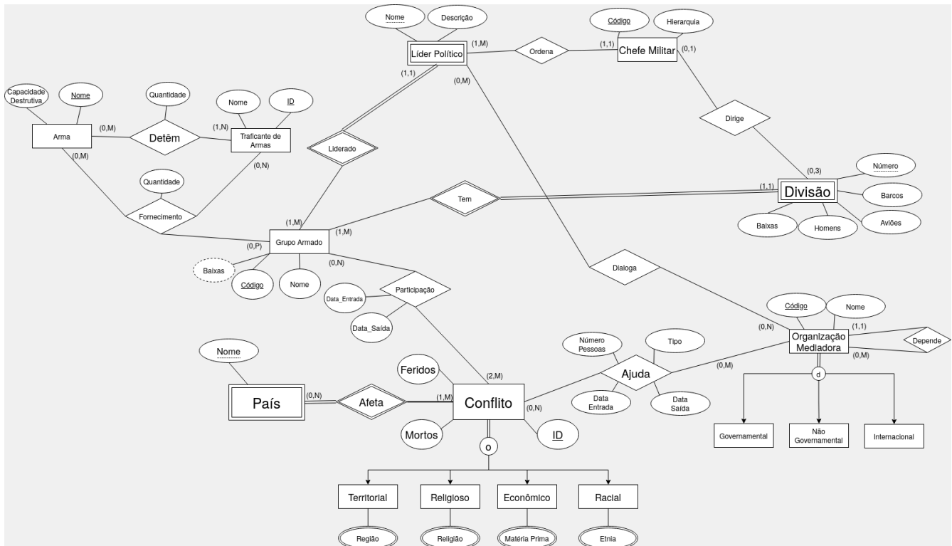
Figura 1: Diagrama de Entidade Relacionamento Estendido
