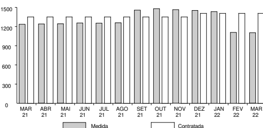
Demanda Fora da Ponta (Medida x Contratada) em kW
