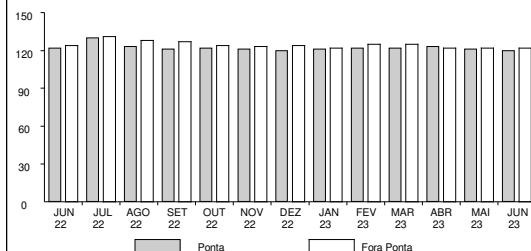
Demanda Medido (Ponta e Fora Ponta) em kW
