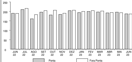
Uso Fio Medido (Ponta e Fora Ponta) em kW
