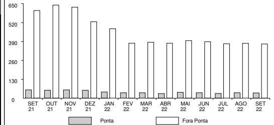
Consumo Ativo Faturado (Ponta e Fora Ponta) em MWh
