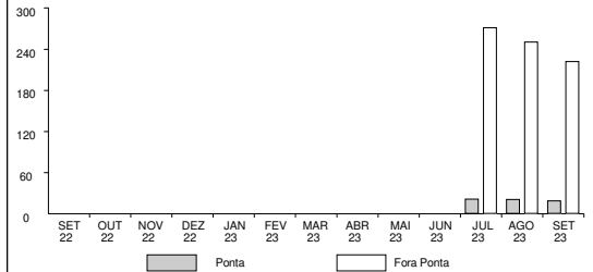
Uso Encargo Faturado (Ponta e Fora Ponta) em MWh
