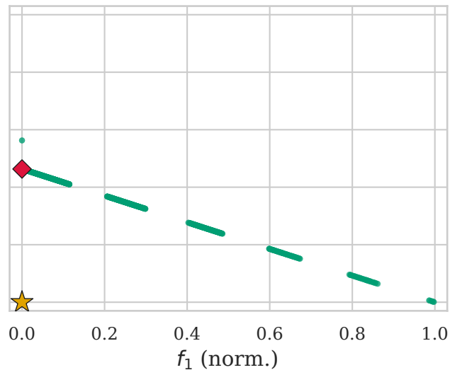
PI-NSGA-II
