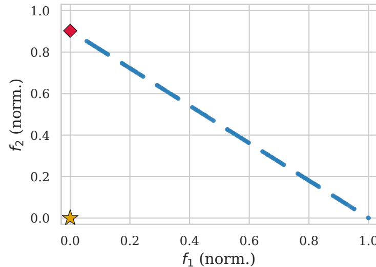
NSGA-II
