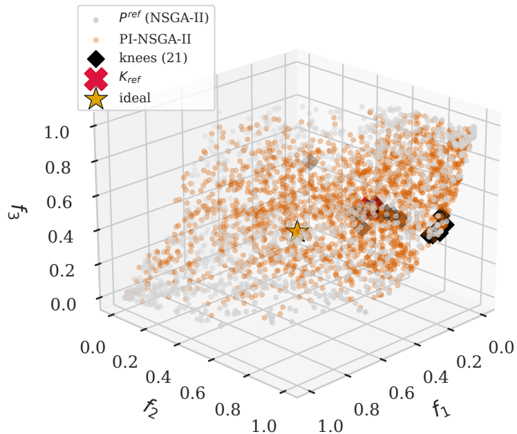
PI-NSGA-II
