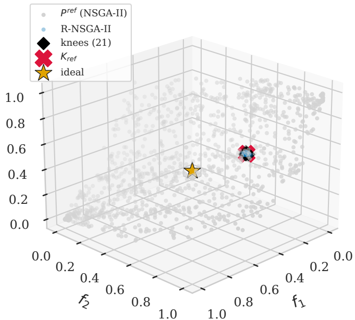
R-NSGA-II
