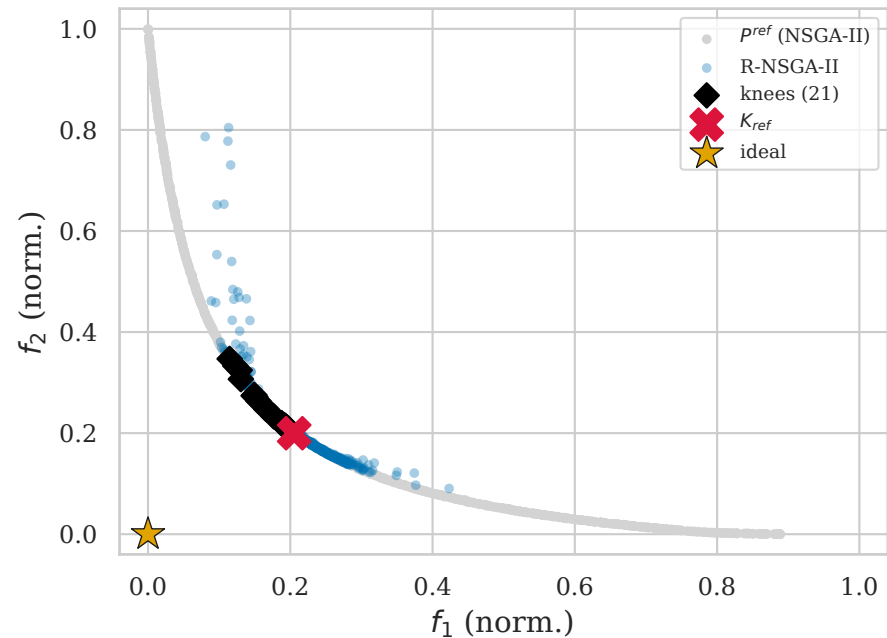
R-NSGA-II
