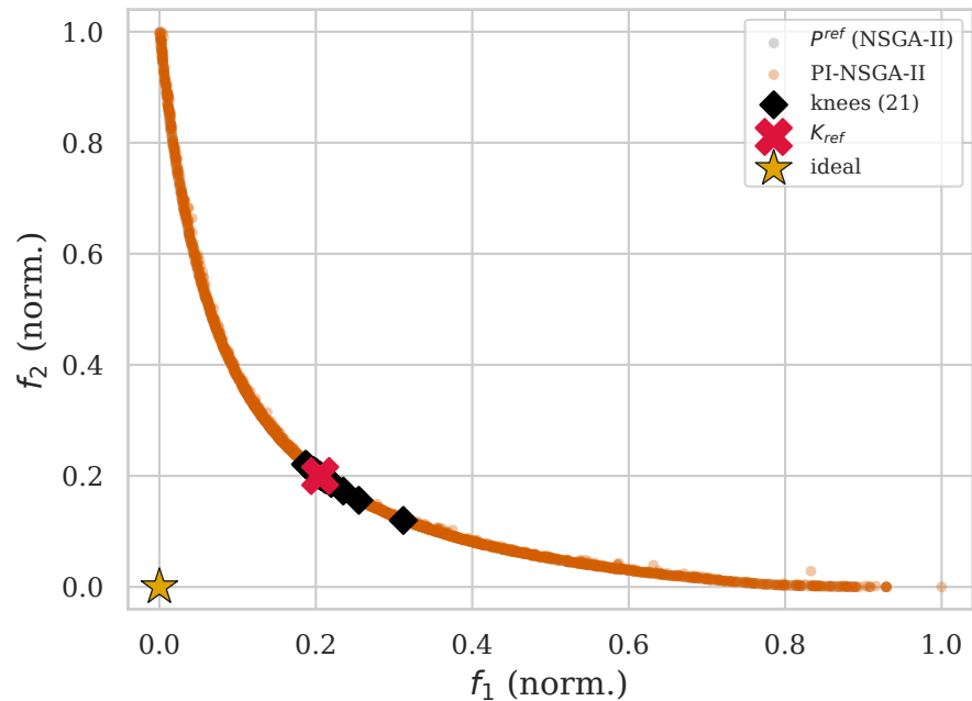
PI-NSGA-II
