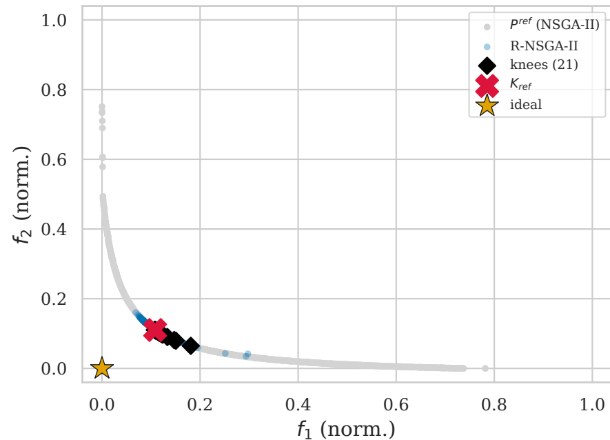
R-NSGA-II
