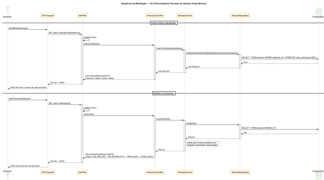
Figura 15 - Realizacao UC-05 Acompanhar Processo de Adoacao
