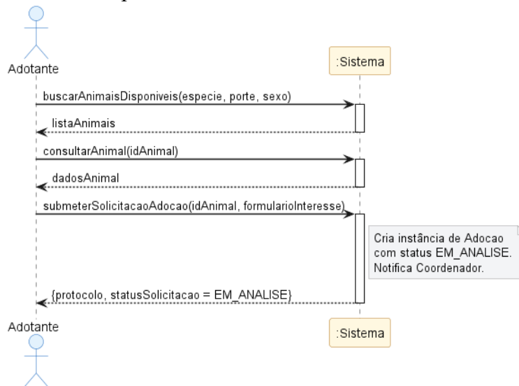
Figura 2 - SSD UC-01 Solicitar Adocao
