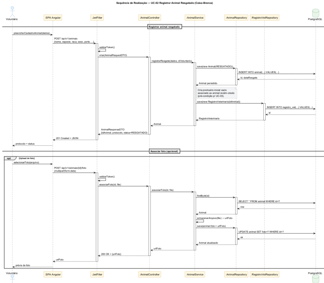
Figura 12 - Realização UC-02 Registrar Animal Resgatado
