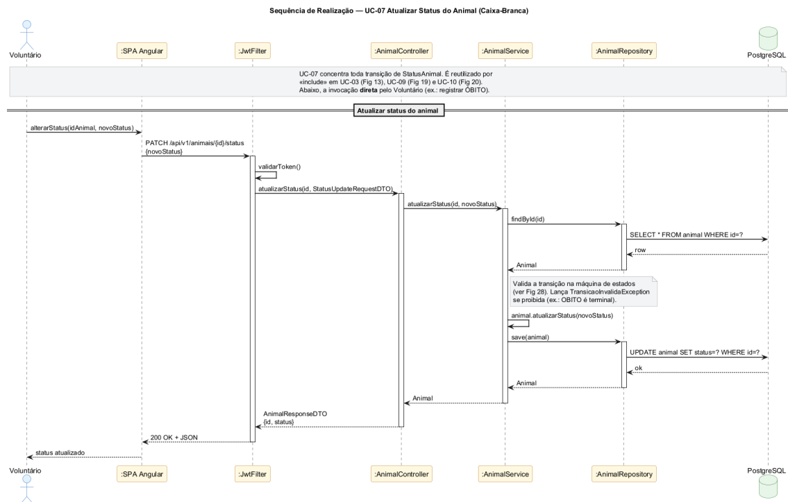
Figura 17 - Realizacao UC-07 Atualizar Status do Animal
