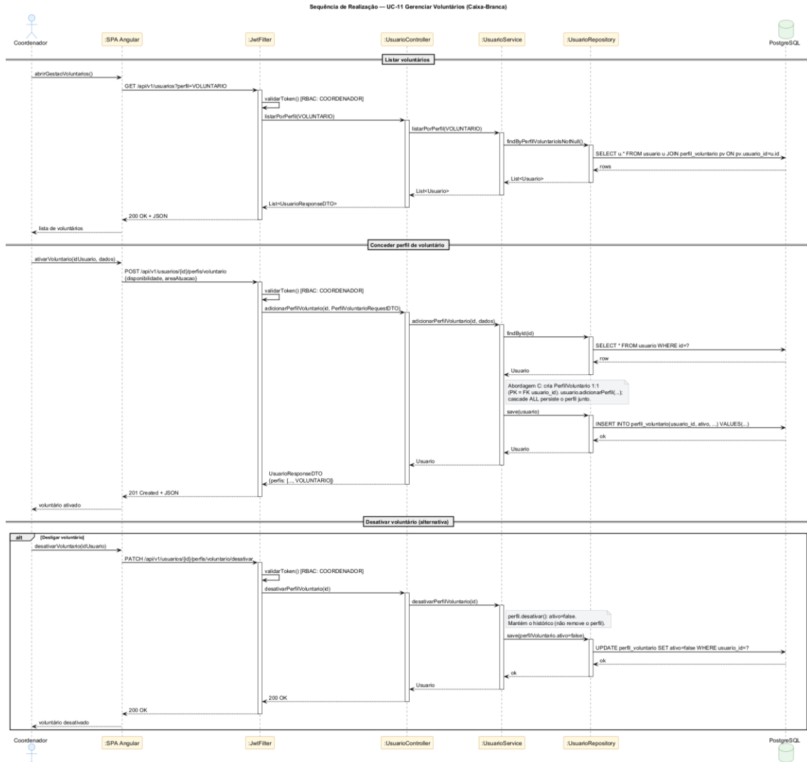
Figura 21 - Realização UC-11 Gerenciar Voluntários
