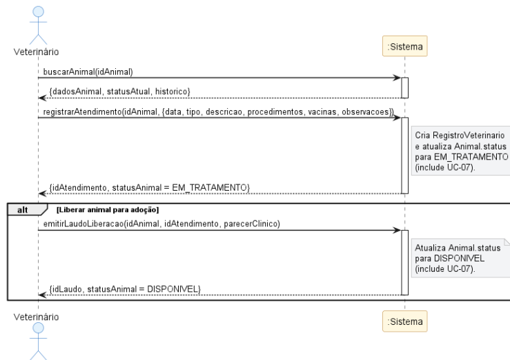
Figura 4 - SSD UC-03 Registrar Atendimento Veterinario
