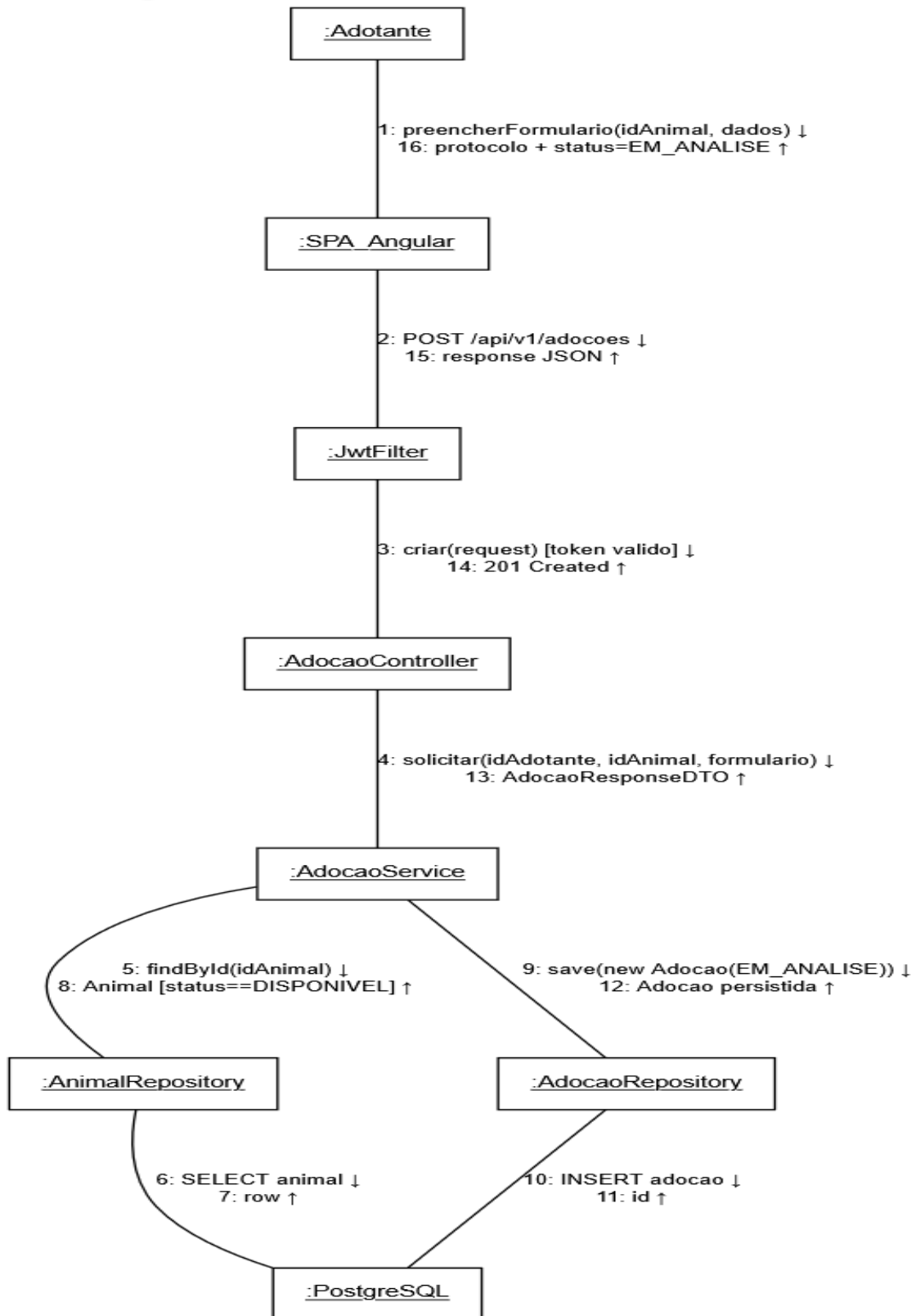
Figura 25 - Comunicacao UC-01 Solicitar Adocao
