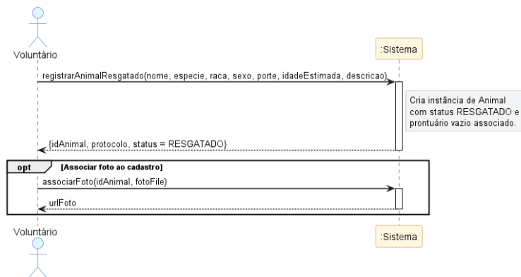
Figura 3 - SSD UC-02 Registrar Animal Resgatado
