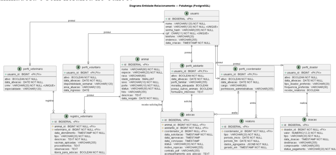
Figura 29 - Diagrama Entidade-Relacionamento do PataAmiga (PostgreSQL)
