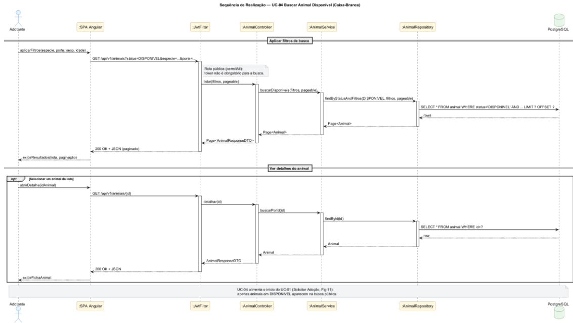
Figura 14 - Realizacao UC-04 Buscar Animal Disponível
