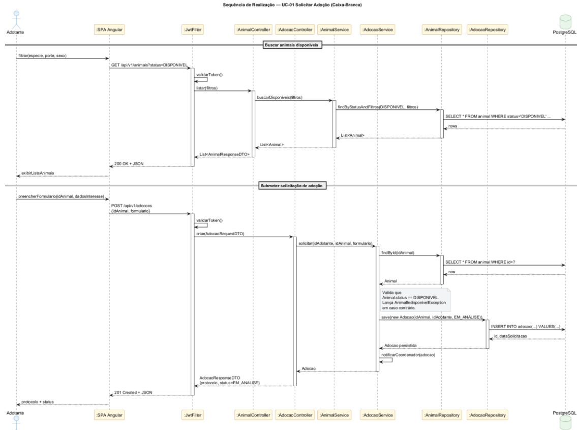
Figura 11 - Realizacao UC-01 Solicitar Adocao
