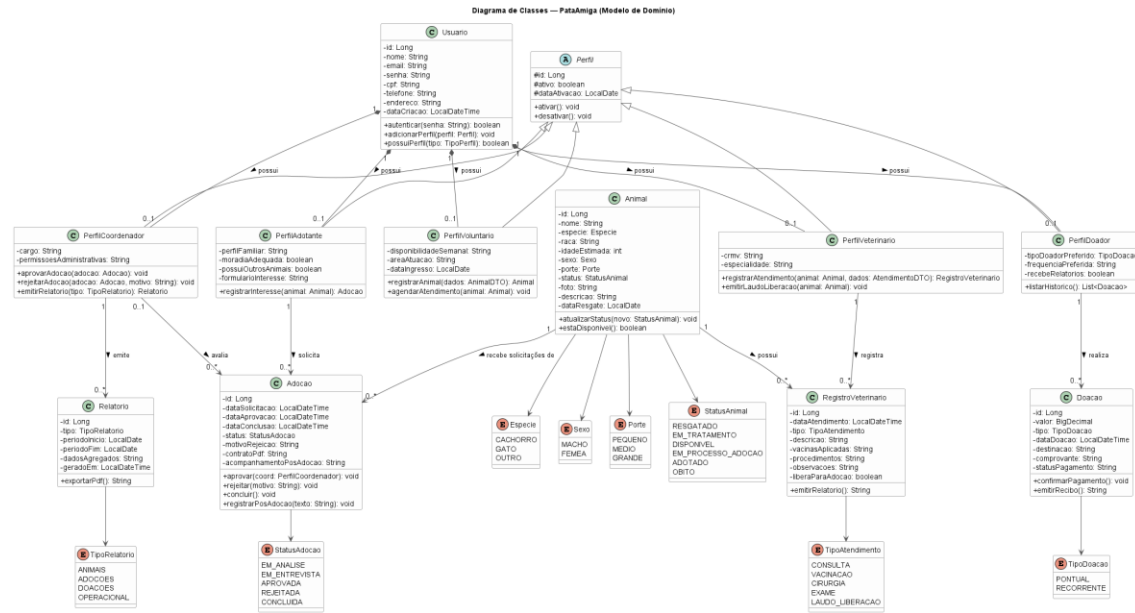
Figura 9 - Diagrama de Classes do Modelo de Domínio do PataAmiga
