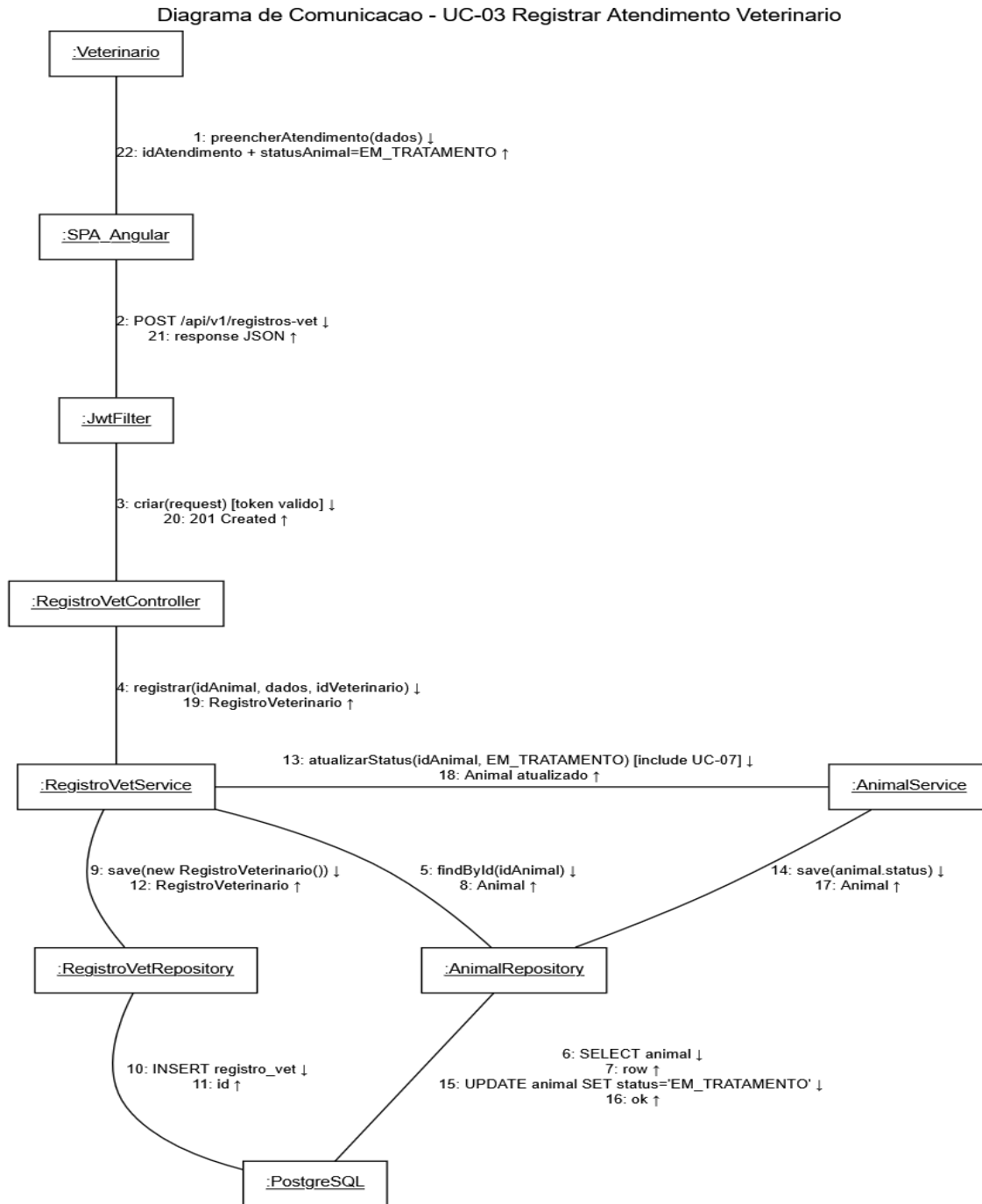
Figura 27 - Comunicacao UC-03 Registrar Atendimento Veterinario
