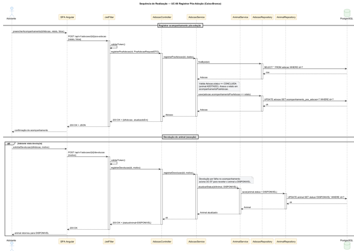
Figura 16 - Realizacao UC-06 Registrar Pos-Adocao
