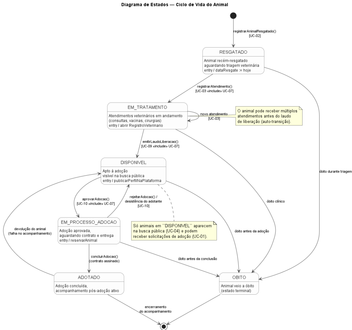
Figura 28 - Diagrama de Estados: Ciclo de Vida do Animal
