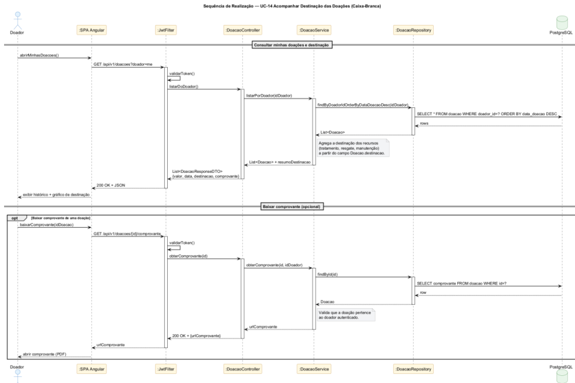
Figura 24 - Realizacao UC-14 Acompanhar Destinação das Doacoes
