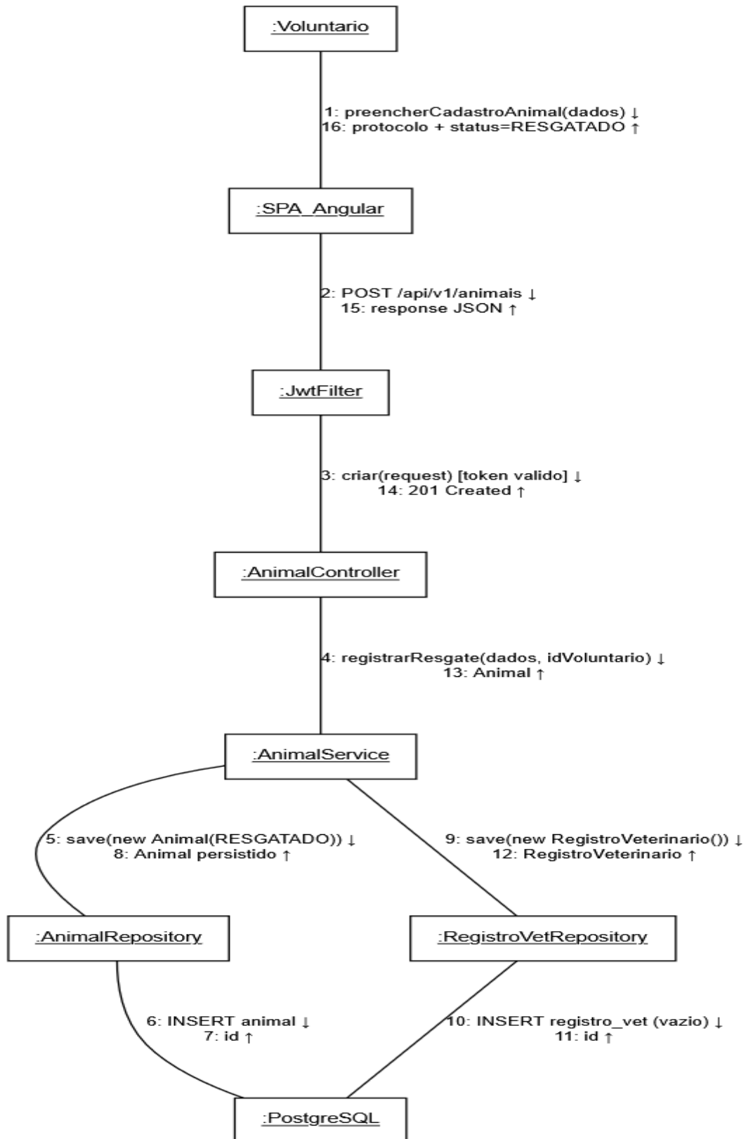
Figura 26 - Comunicacao UC-02 Registrar Animal Resgatado
