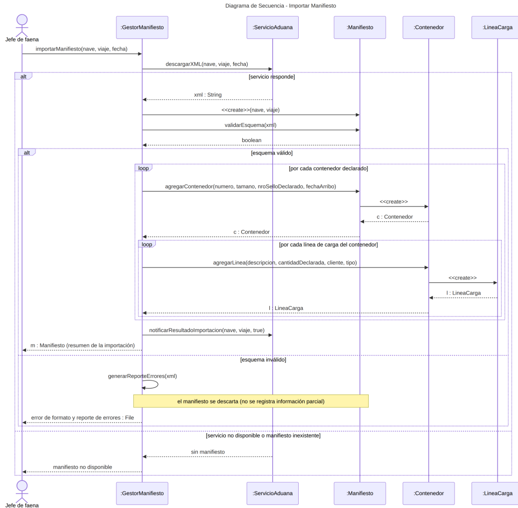
Figura 13: Diagrama de secuencia - Importar manifiesto.
