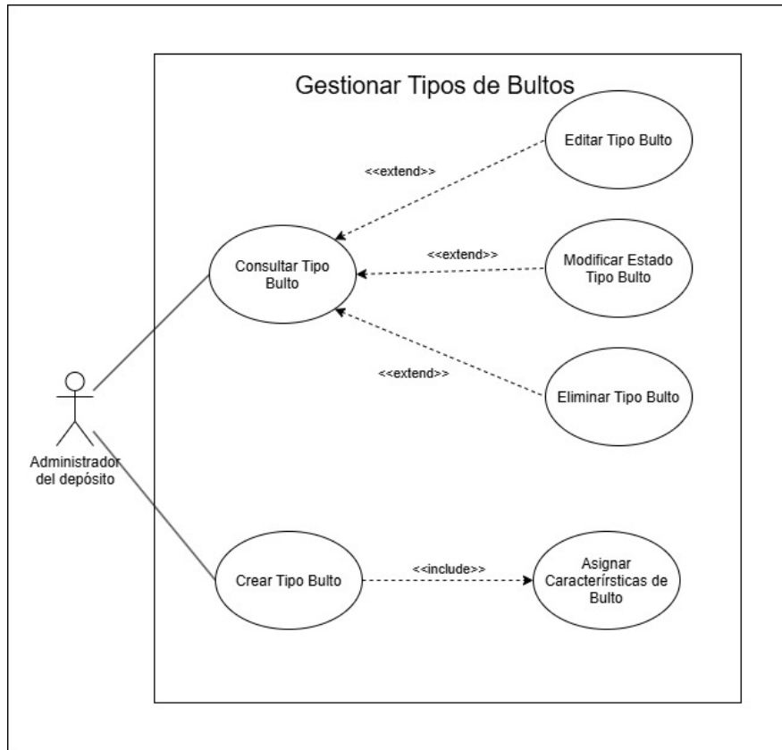
Figura 4: Gestionar tipos de bultos - Diagrama expandido.
