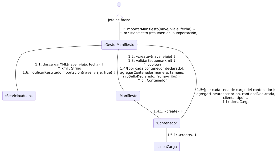
Figura 17: Diagrama de colaboración - Importar manifiesto.
