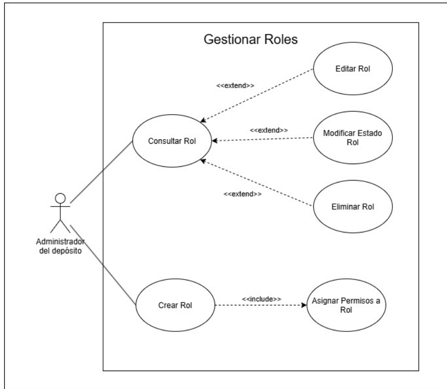
Figura 3: Gestionar roles - Diagrama expandido.
