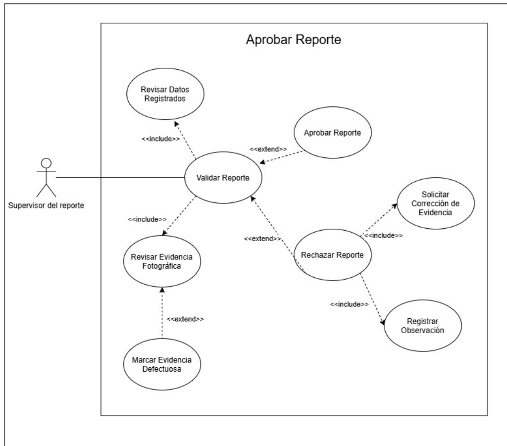
Figura 11: Aprobar reporte - Diagrama expandido.
