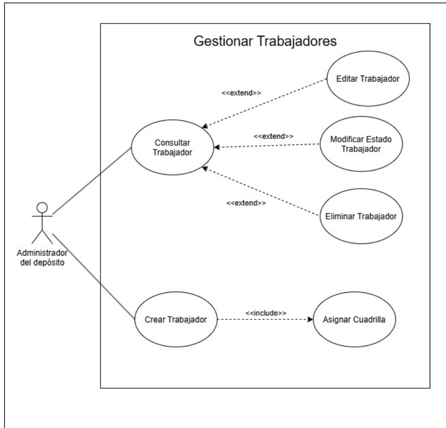
Figura 6: Gestionar trabajadores - Diagrama expandido.
