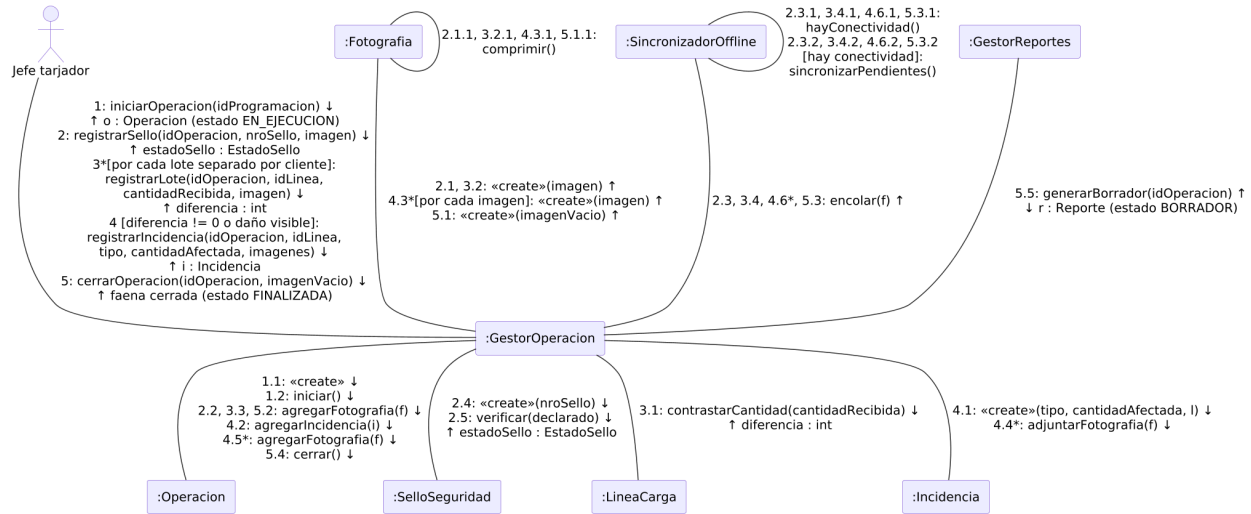
Figura 19: Diagrama de colaboración - Registrar datos de operación.
