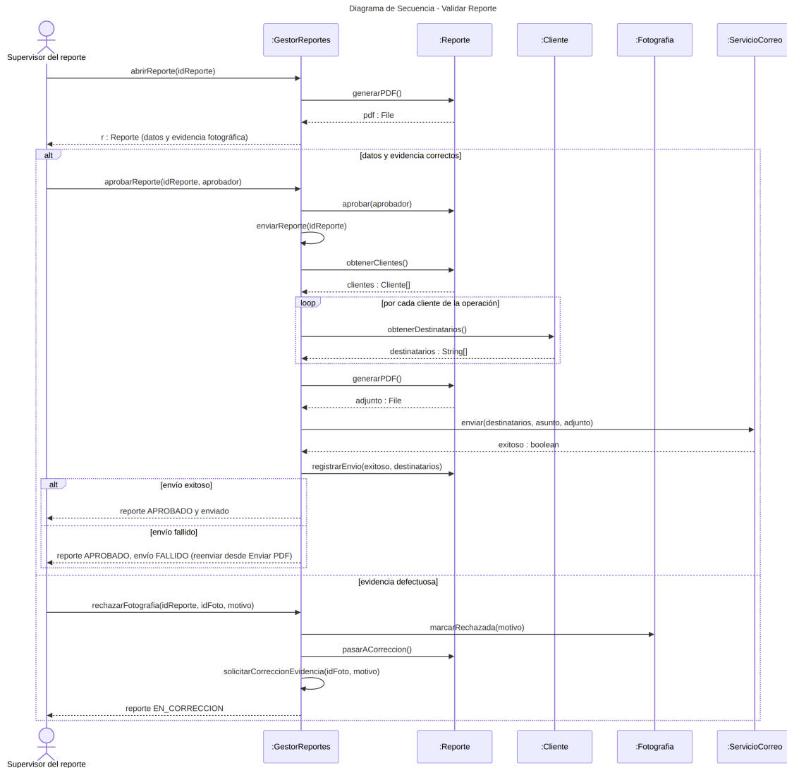
Figura 16: Diagrama de secuencia - Validar reporte.
