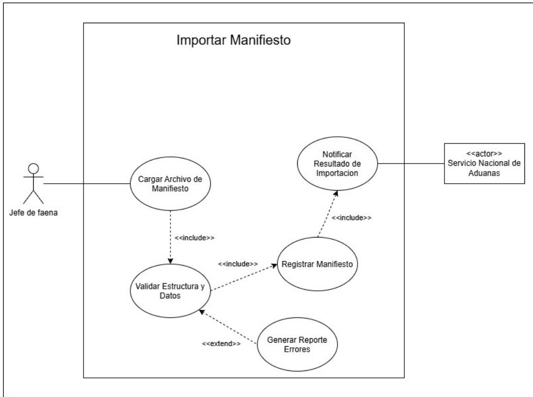
Figura 7: Importar manifiesto - Diagrama expandido.
