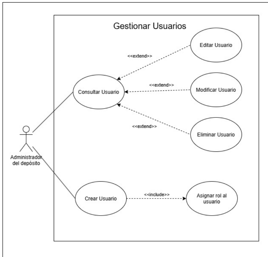
Figura 2: Gestionar usuarios - Diagrama expandido.
