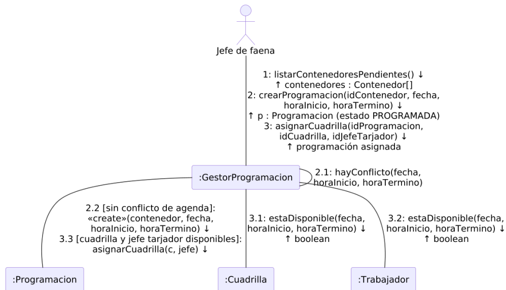
Figura 18: Diagrama de colaboración - Crear programación.
