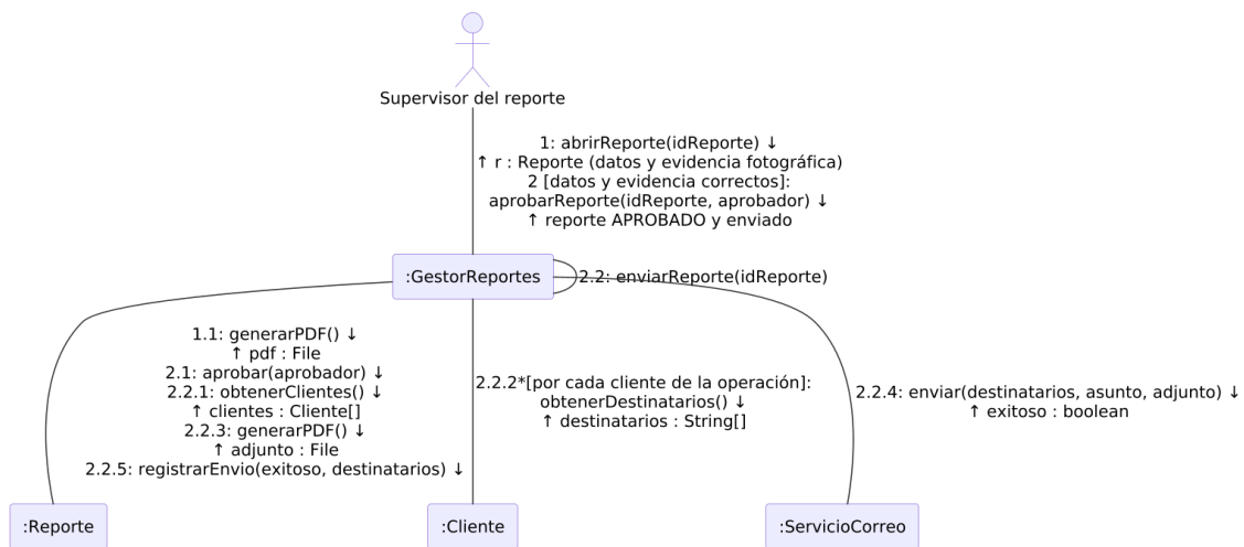
Figura 20: Diagrama de colaboración - Validar reporte (curso de aprobación y envío).
