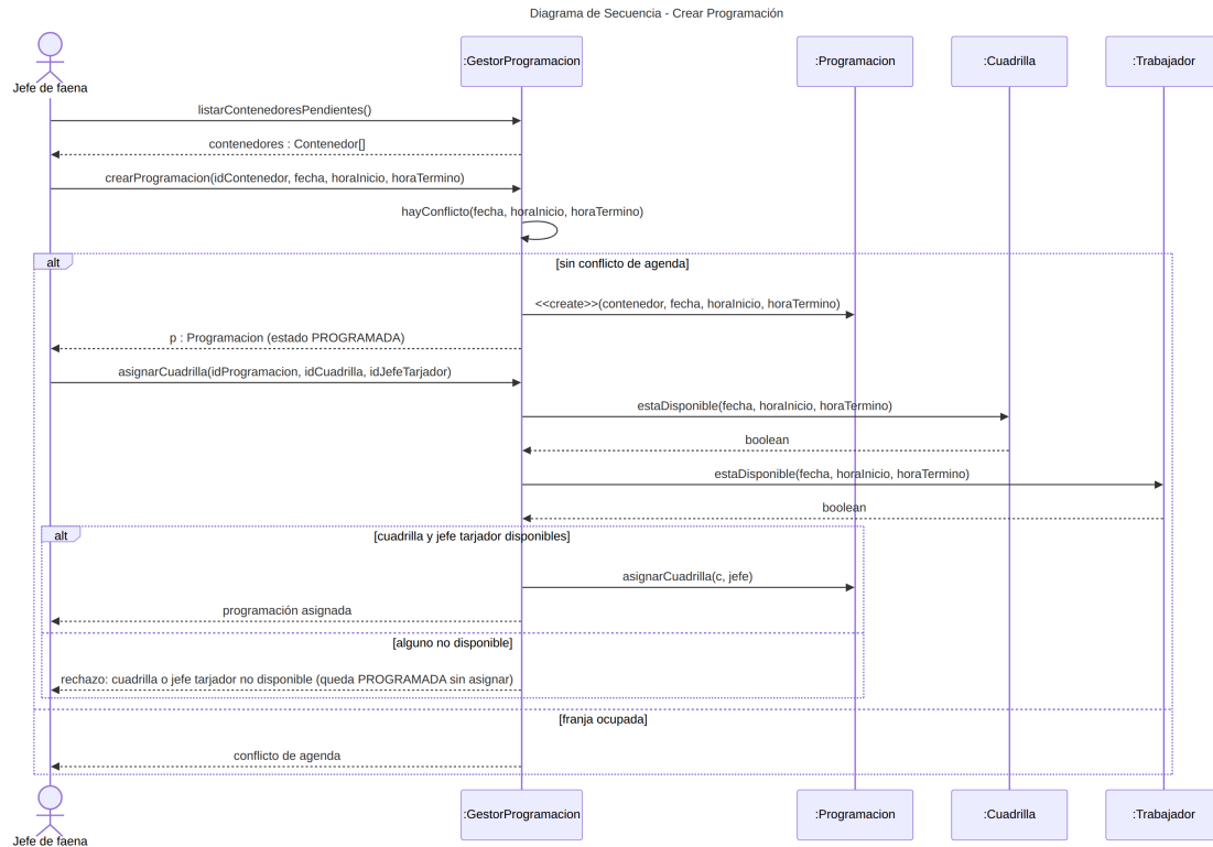
Figura 14: Diagrama de secuencia - Crear programación.
