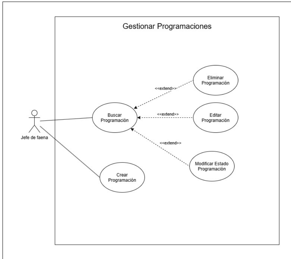
Figura 8: Gestionar programaciones - Diagrama expandido.
