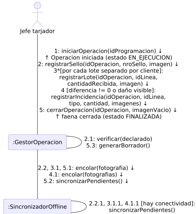
Figura 19: Diagrama de colaboración - Registrar datos de operación.
