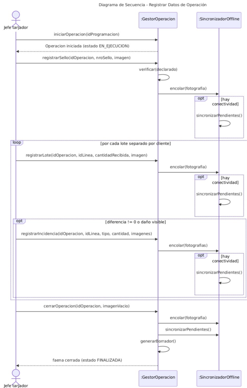
Figura 15: Diagrama de secuencia - Registrar datos de operación.
