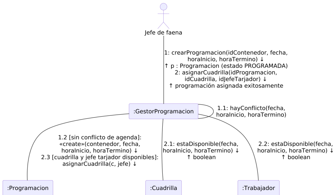
Figura 18: Diagrama de colaboración - Crear programación.
