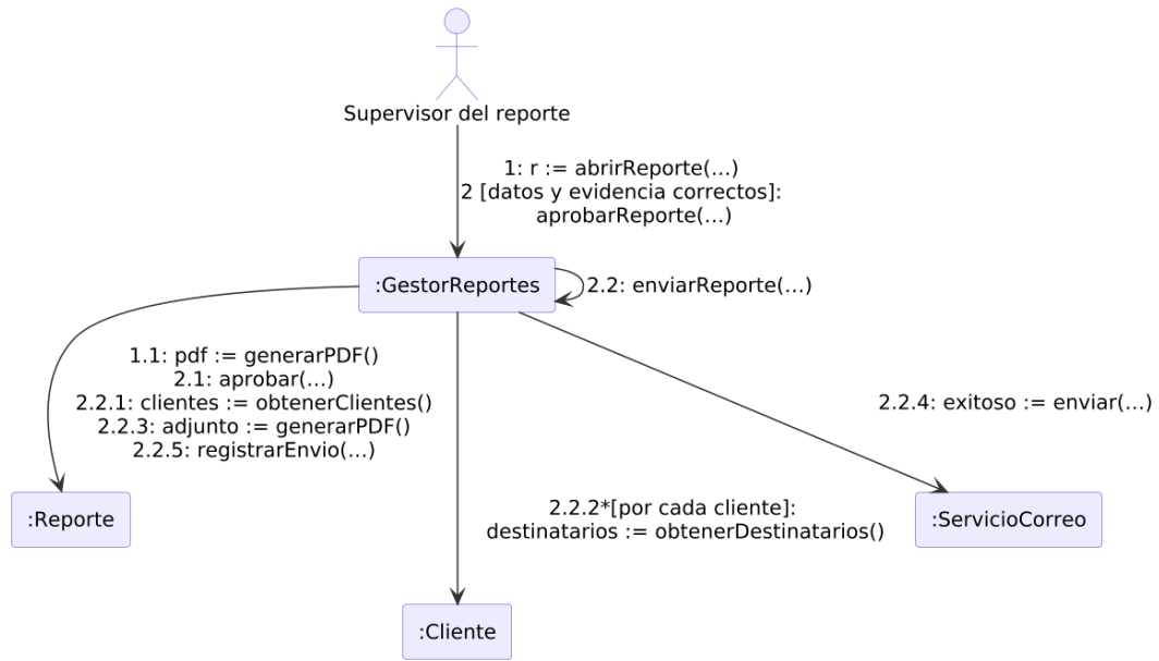
Figura 20: Diagrama de colaboración - Validar reporte (curso de aprobación y envío).
