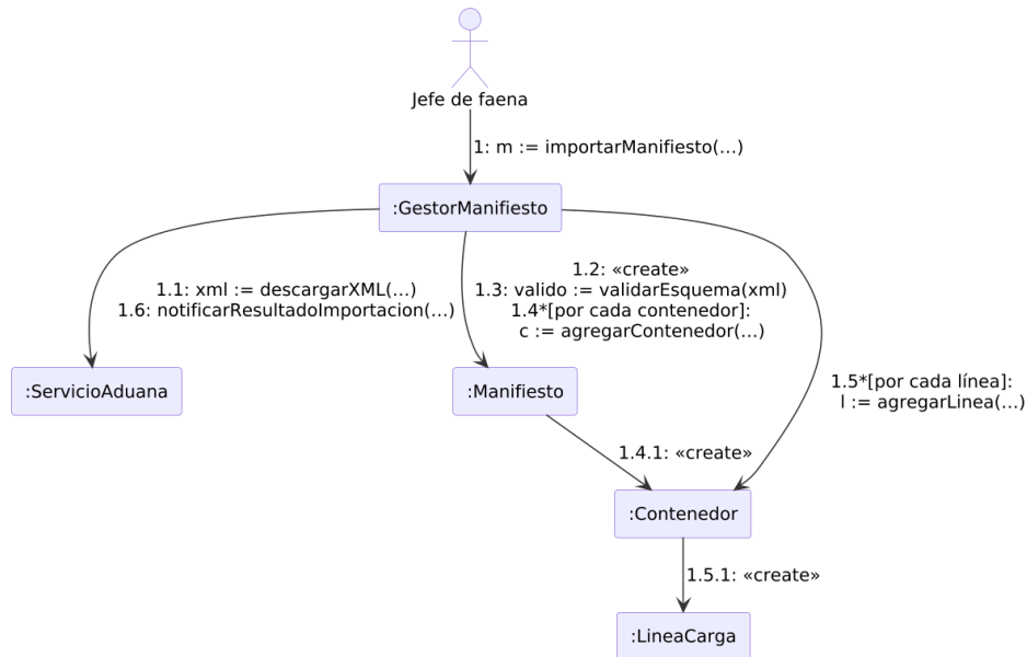
Figura 17: Diagrama de colaboración - Importar manifiesto.
