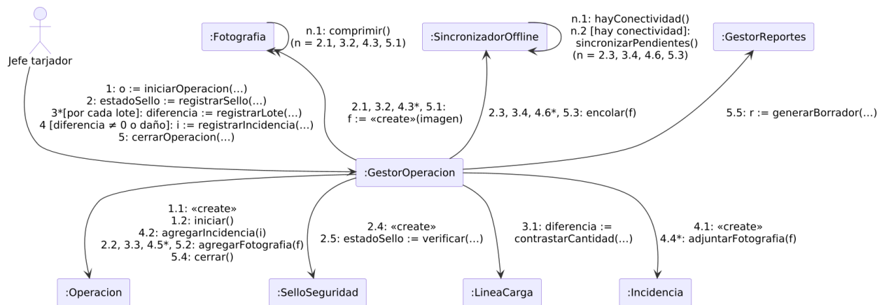
Figura 19: Diagrama de colaboración - Registrar datos de operación.
