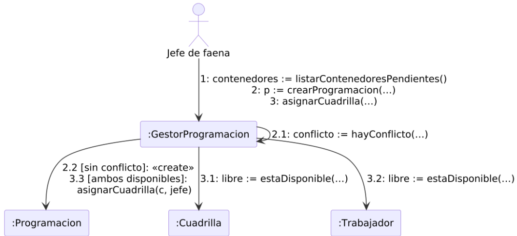
Figura 18: Diagrama de colaboración - Crear programación.
