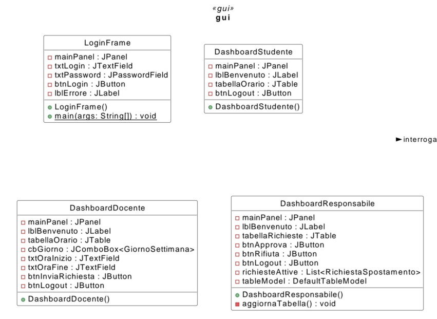
Figura 6: Ingegnerizzazione dello strato Boundary (Interfaccia Grafica).
