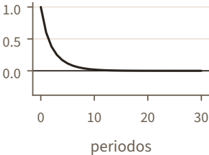
reales
