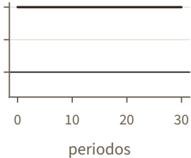
raíz unitaria
