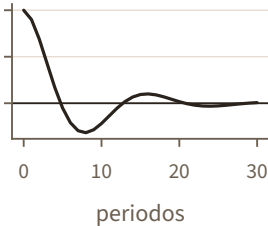
complejos
