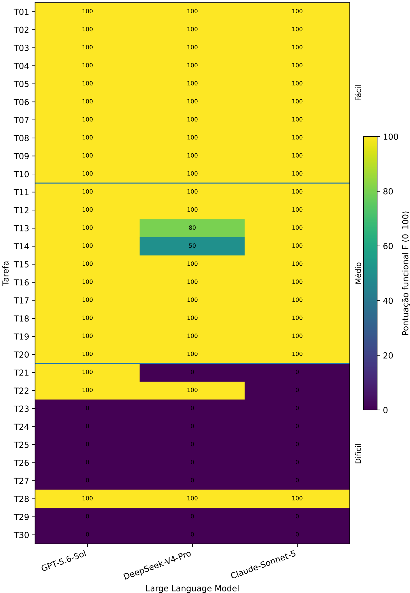
Desempenho funcional por tarefa e modelo
