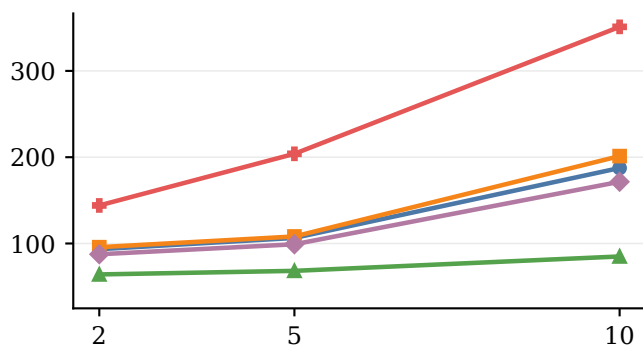
MMLU
