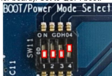
Figure 21. RZ/G2L-EVK & RZ/V2L-EVK QSPI boot mode
