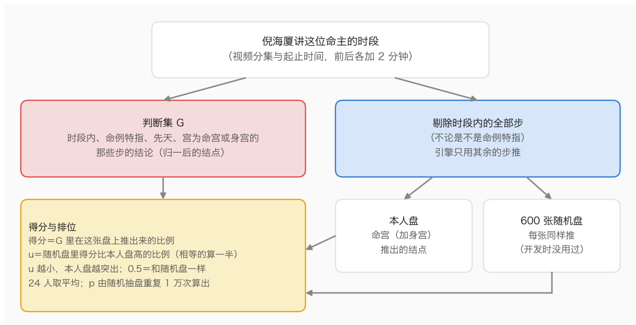
S图 8 主检验的设计
