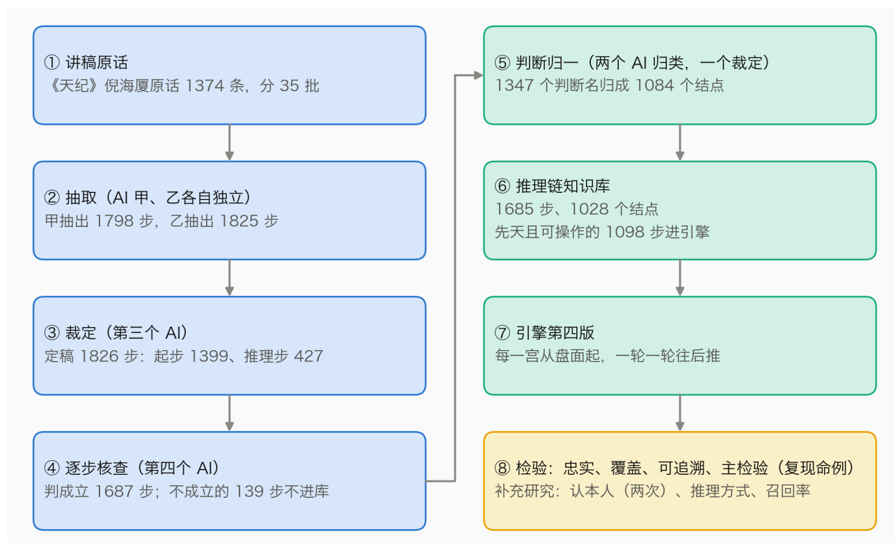
图 1 全文流程
