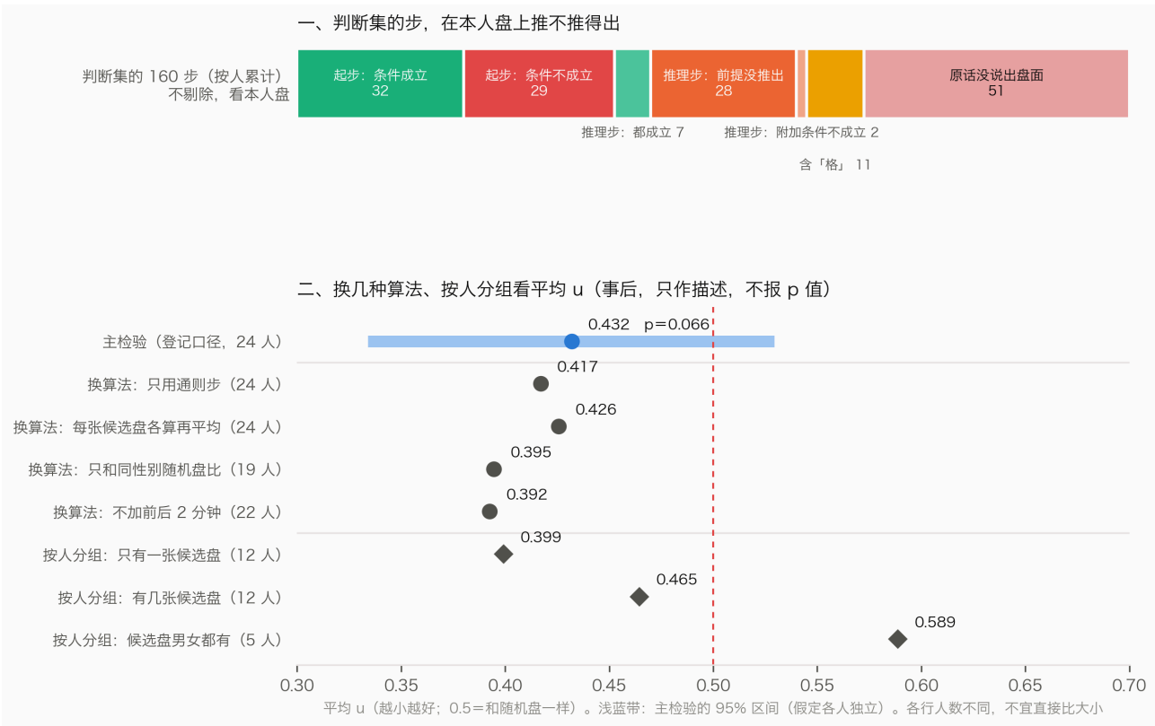
S图 10 内审后的补充分析 (只作描述)：判断集的步在本人盘上推不推得出 (上，按人累计)；换几种算法、按人分组看平均 u (下)
