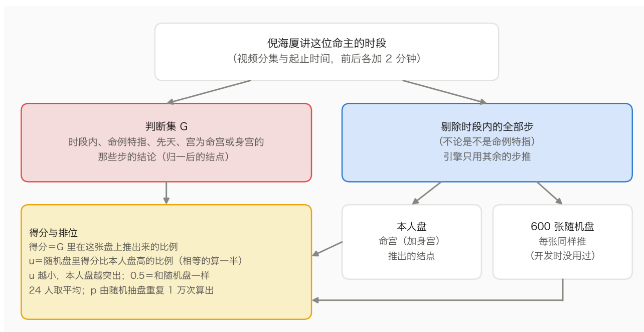
S图 8 主检验的设计
