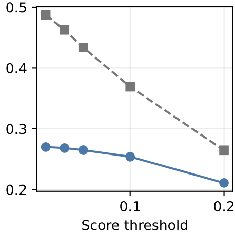
OWL-ViT
