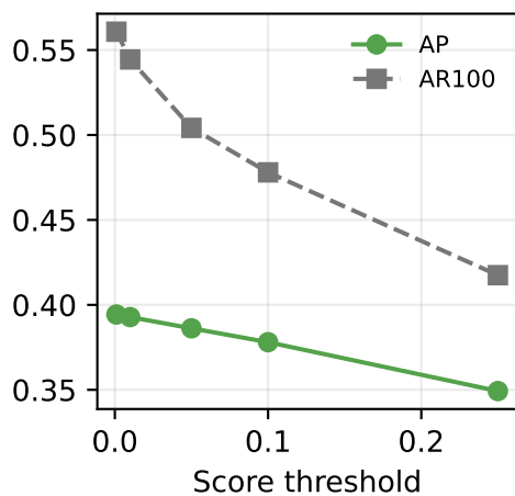
YOLO-World
