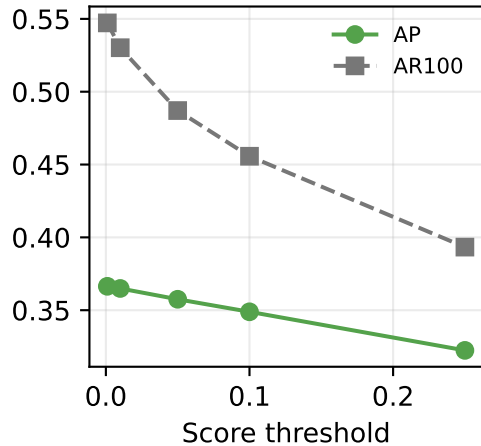
YOLO-World
