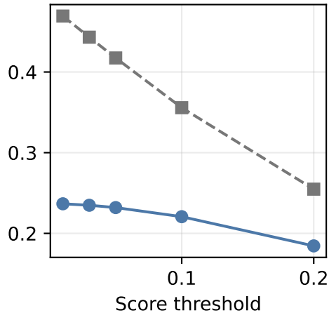
OWL-ViT
