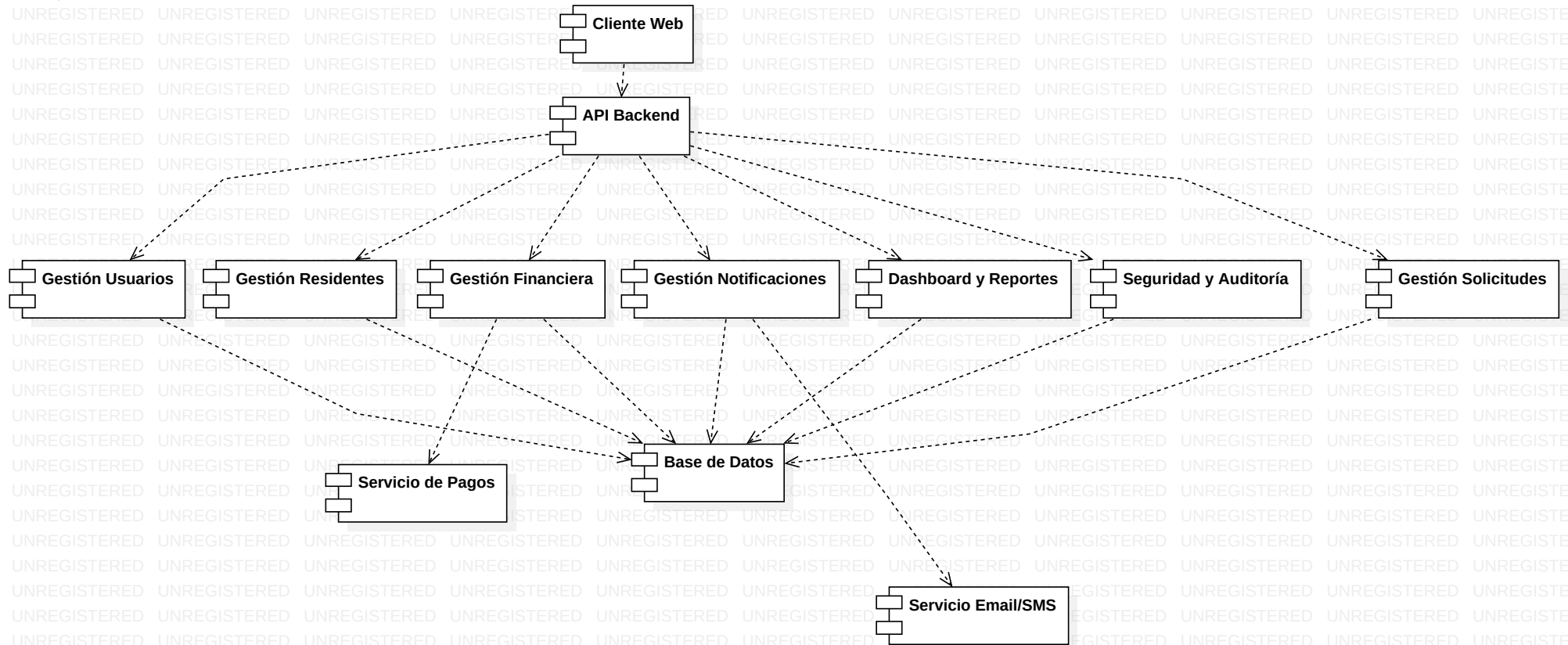
Diagrama de Componentes
