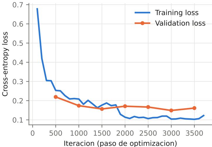
BERT-base · SST-2
