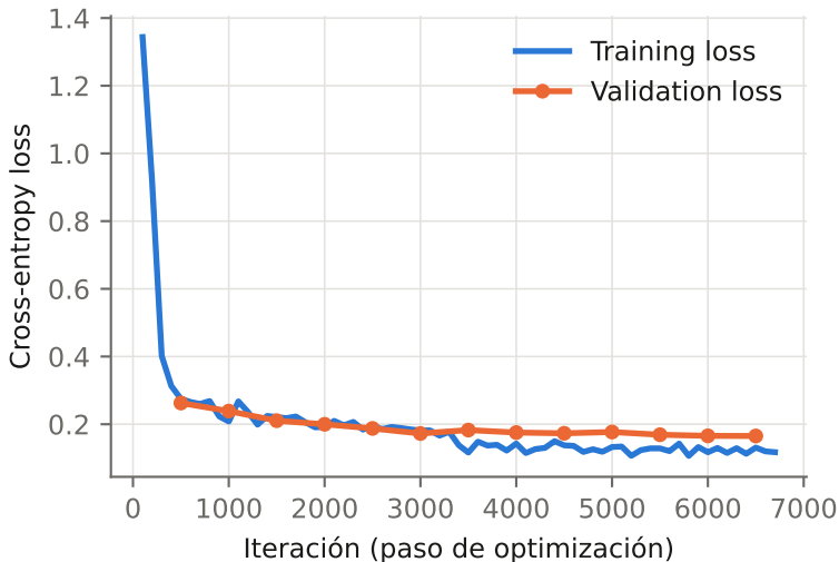
BERT-base · AG News
