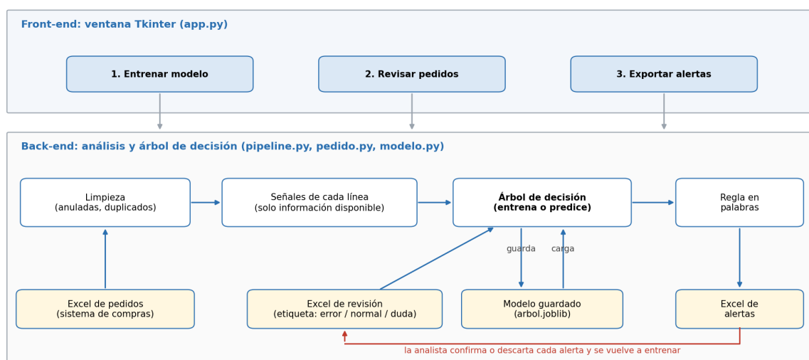
Figura 14: Arquitectura del software. La ventana (arriba) llama al análisis (abajo); el árbol se entrena con el Excel de revisión y se guarda para usarlo en cada revisión.
