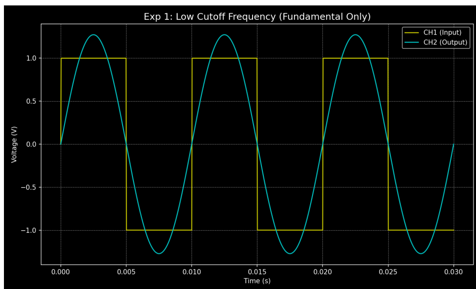
图 1: 低截止频率下的滤波器输出（仅基波）
