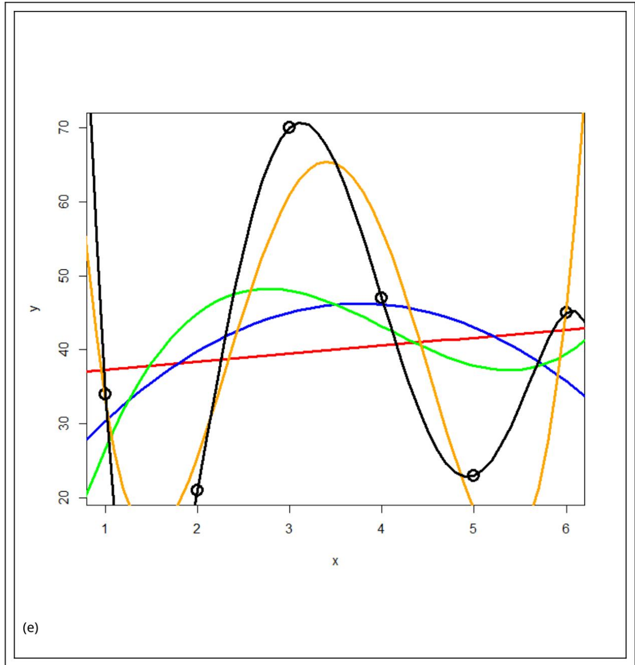
Abbildung 3.3: Overfitting. Die Simulation zeigt, dass die Anpassung des Modells an die Daten immer besser wird, je komplexer ich das Modell mache ( R^2 steigt), in diesem Fall mit der Hinzunahme höherer Polynome.
