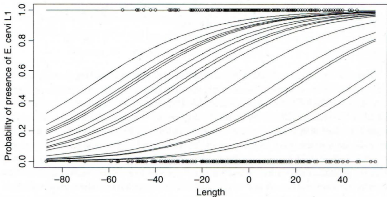
Abb. 6.6. Darstellung der Ergebnisse des GLM-Modells für den Parasiten-Datensatz (aus Zuur et al. 2009).
