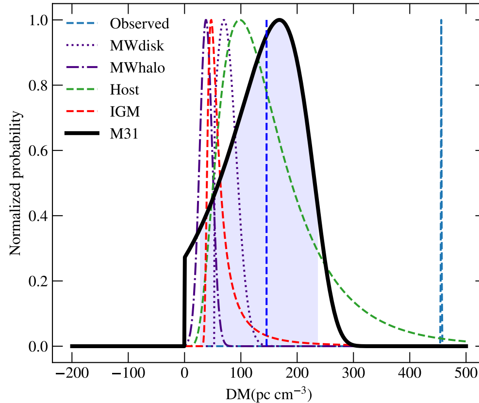
FRB 20230930A
