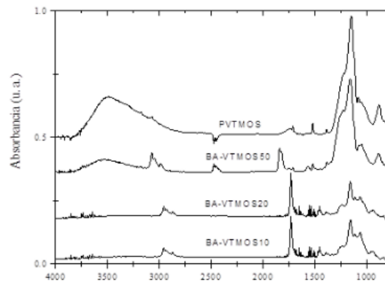
Figura 2: Espectros FTIR de copolímeros BA-VTMOS y sus híbridos obtenidos por sol-gel con TEOS.
