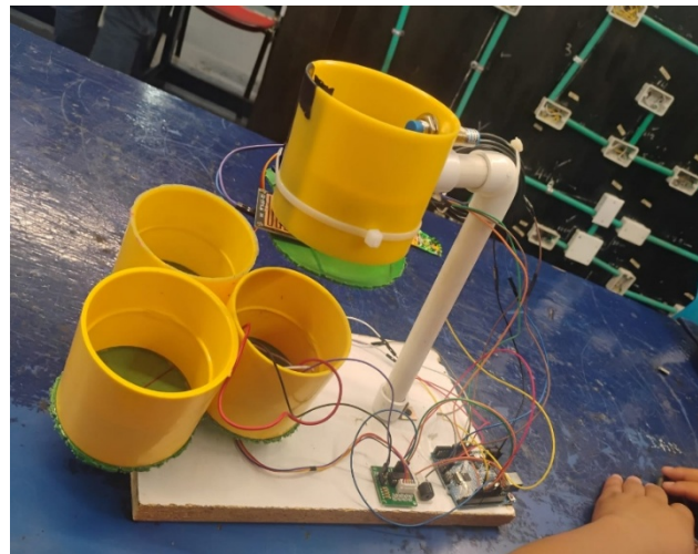
• Figura 1 Prototipo funcional inteligente de separación de residuos
