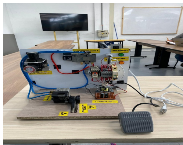
Figura 1 Prototipo funcional para cortes de materiales en la industria de confecciones
