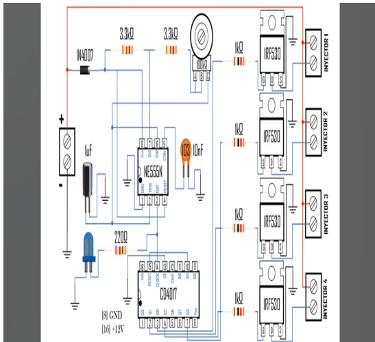
Figura 4: Pulsador de inyectores
