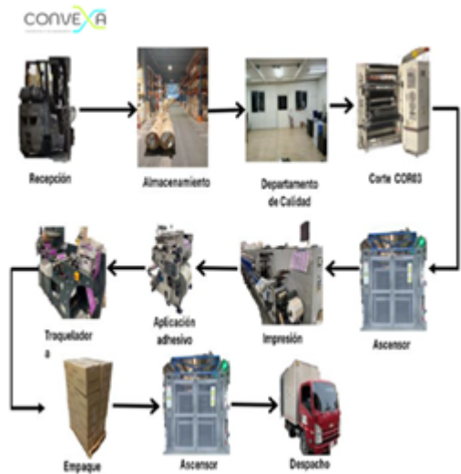
Figura 4 Flujograma del proceso en la empresa Convexa
