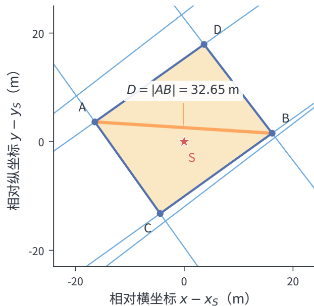
(b) 定位多边形与直径
