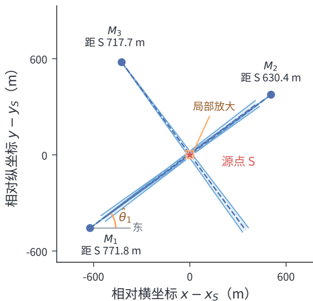
(a) 监测点与测向交会
