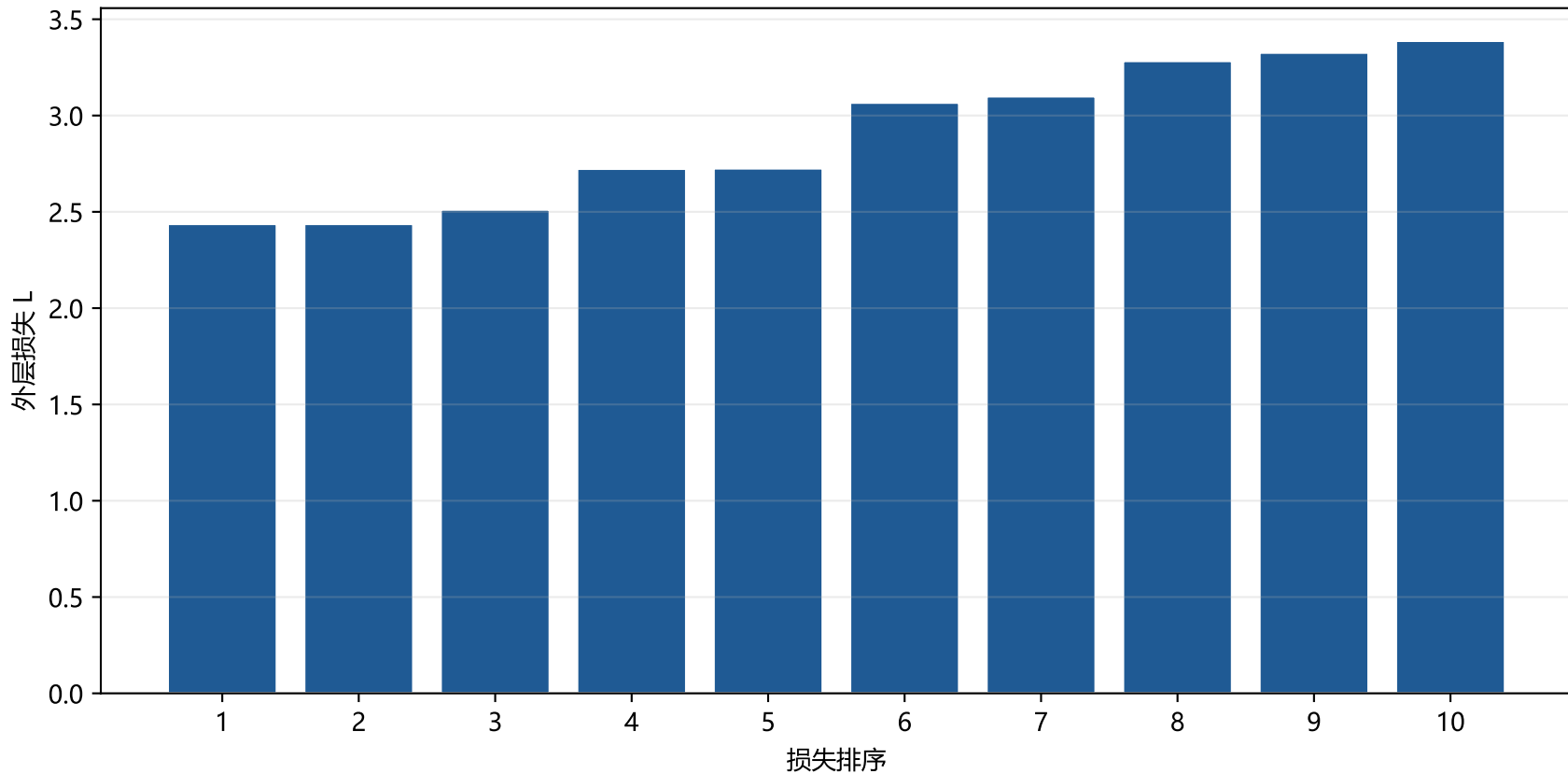
图2-4 蒙特卡洛—权重网格校准的前十组方案
