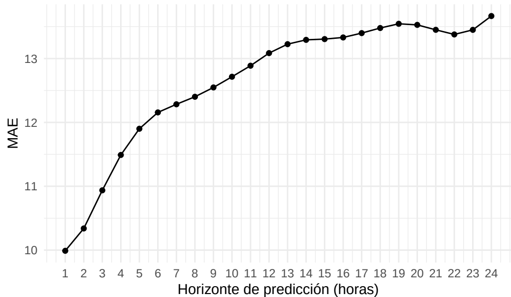
MAE de la ANN según horizonte de predicción
