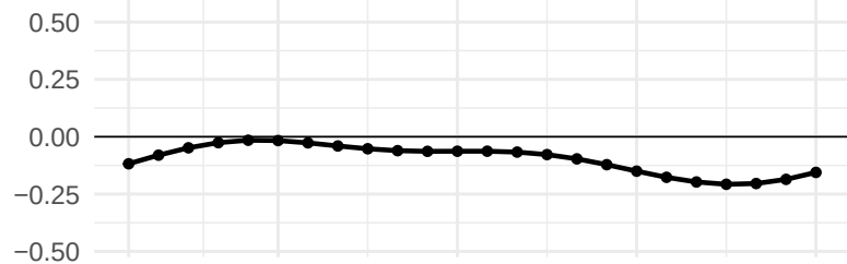
RH
