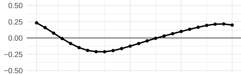
WD_sin
