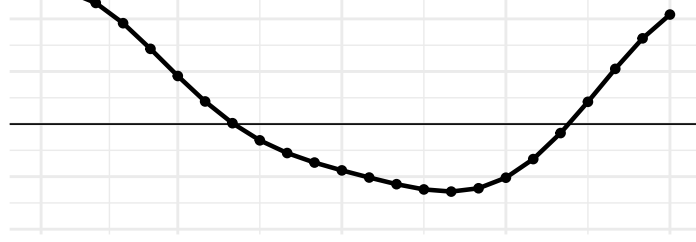
WD_cos
