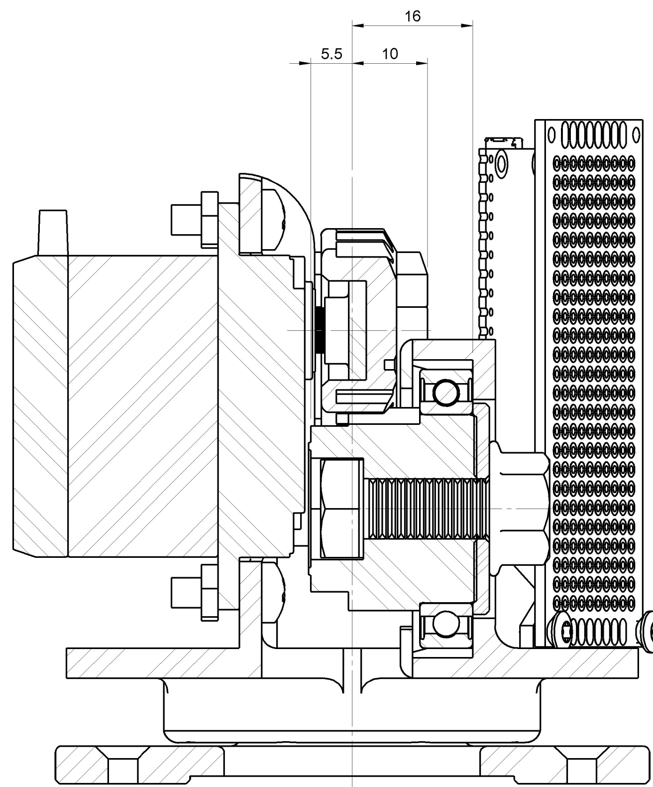
SECTION B-B SCALE: 2:1
